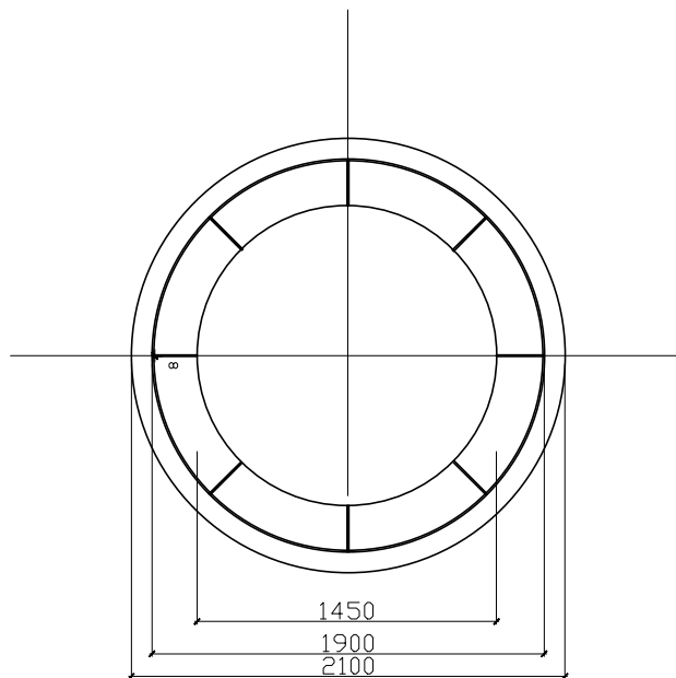
RZUT
