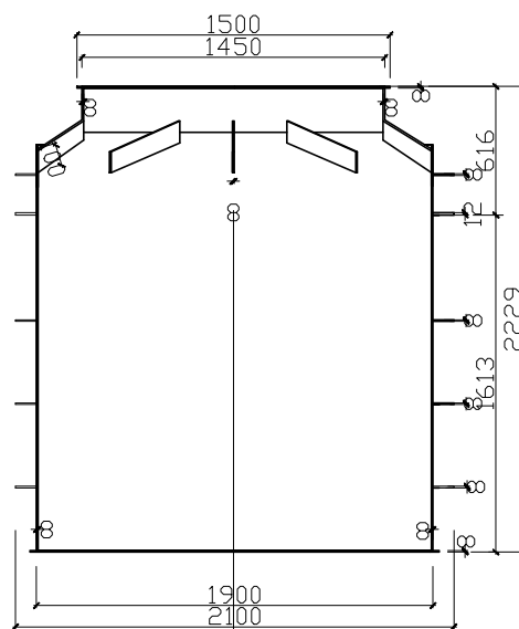
PRZEKRÓJ A-A
