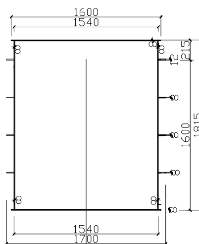
PRZEKRÓJ A-A
